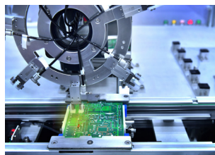
半导体
