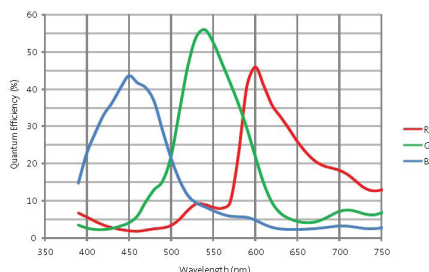
MER-1520-13U3C
