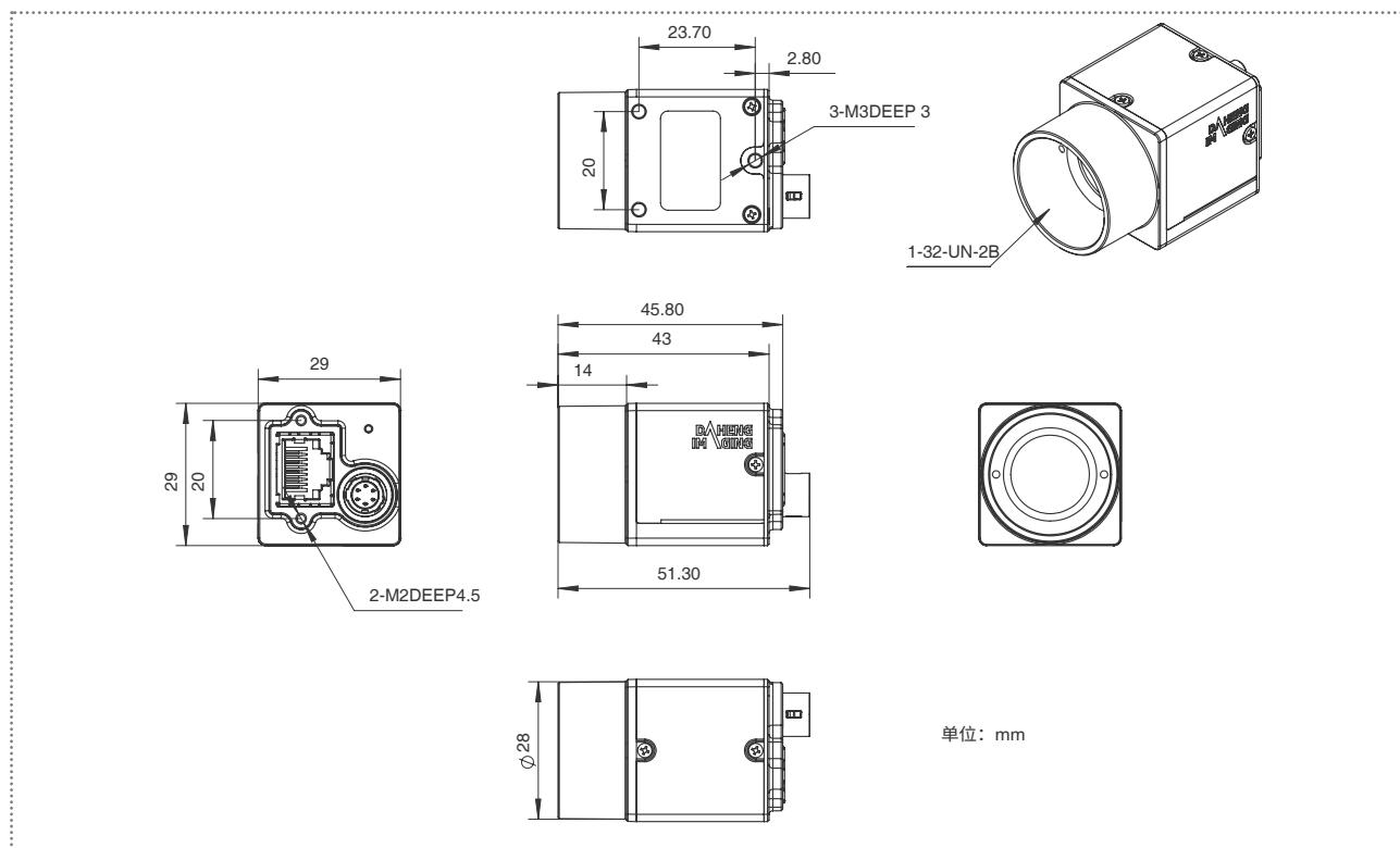
ME2C-160-75GM/C
