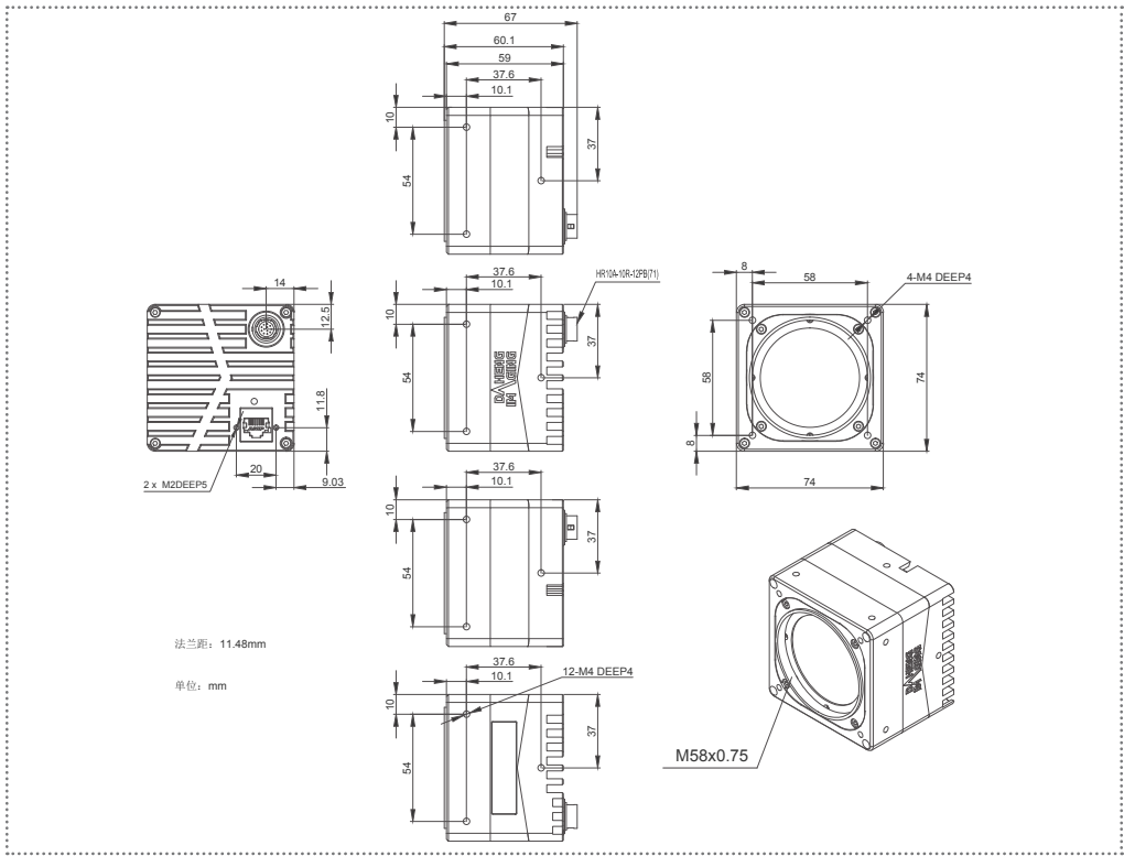
MARS-6500-18GTM/C M58-D1, M58 口 (法兰距 11.48mm)
