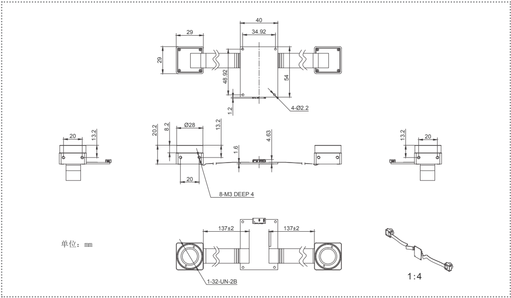
VEN-134-90U3M/C-D, C 口
