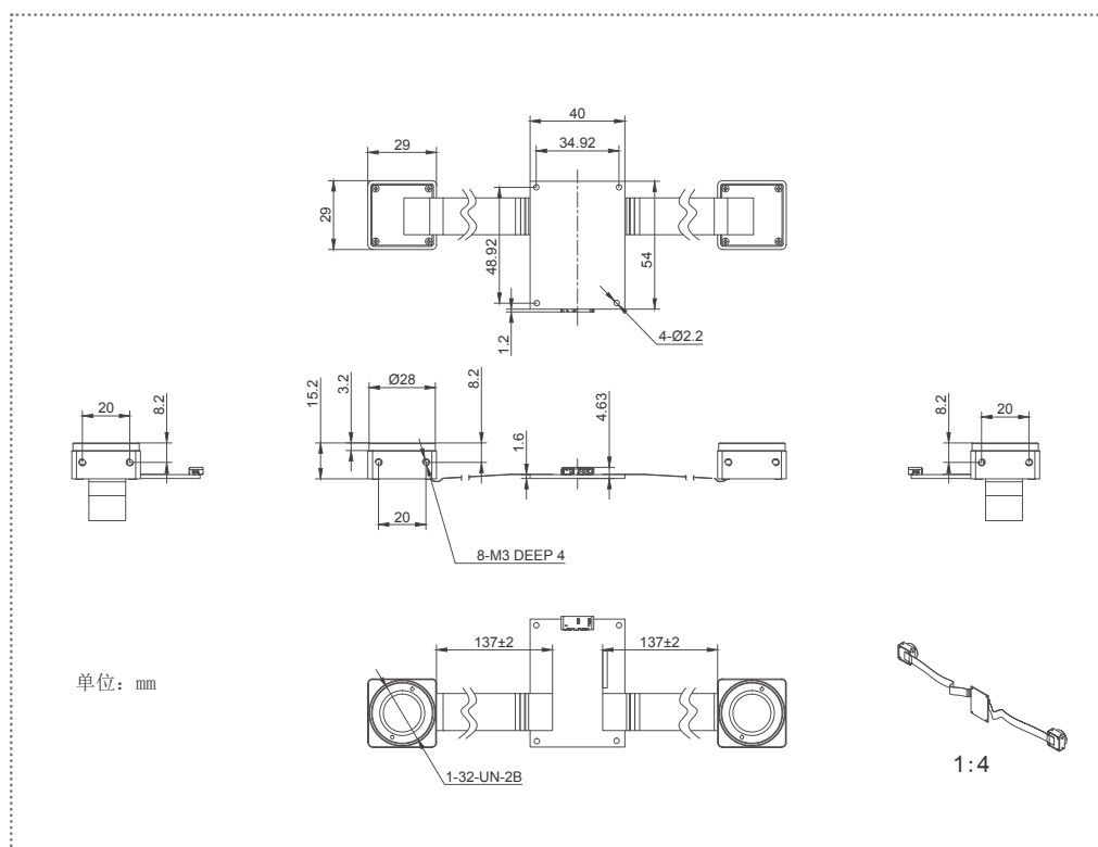
VEN-134-90U3M/C-D, CS 口
