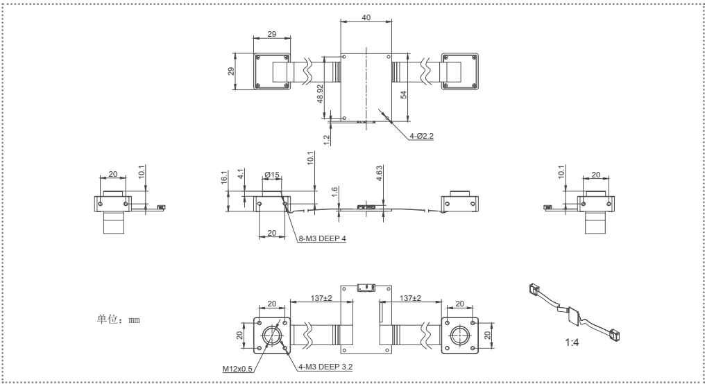
VEN-134-90U3M/C-D, S 口
