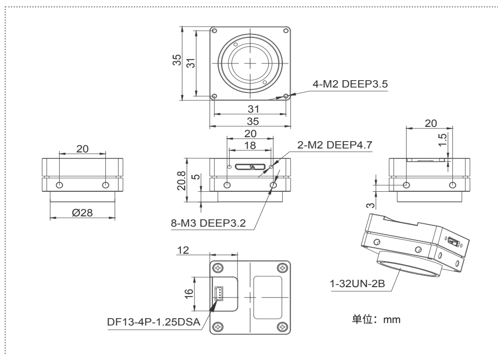
VEN-830-22U3M/C, CS 口
