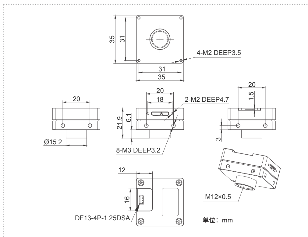
VEN-830-22U3M/C, S 口
