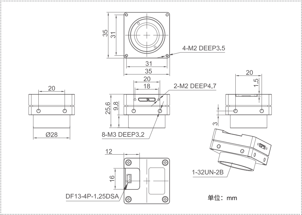
VEN-830-22U3M/C, C 口
