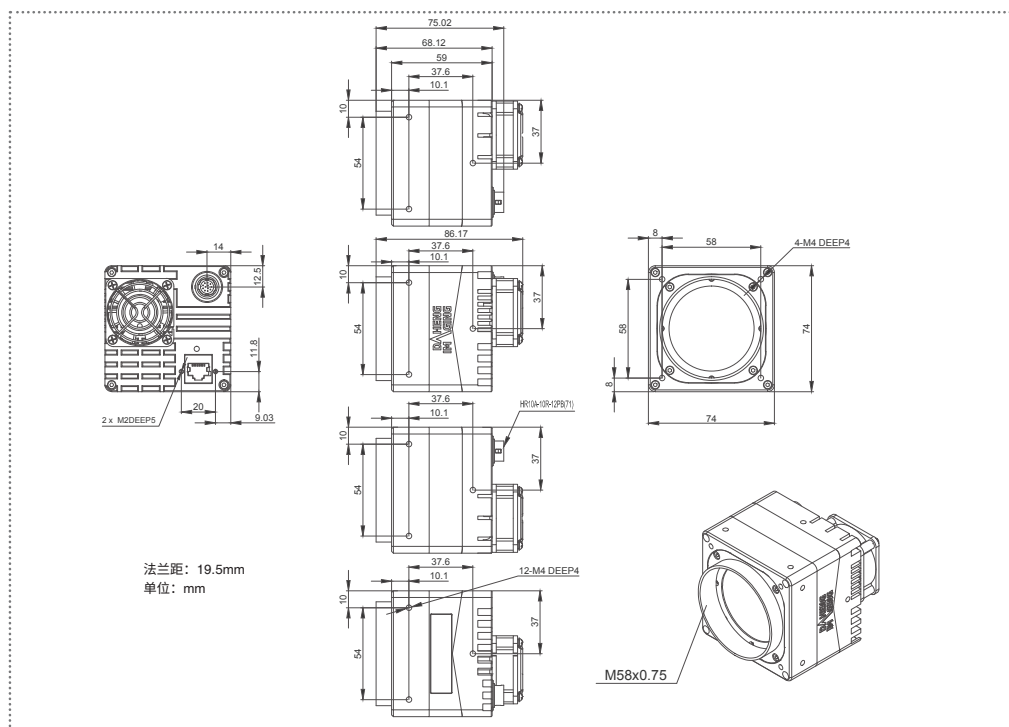
MARS-6500-18GTM/C-NF M58, M58 □ (法兰距 19.5mm)
