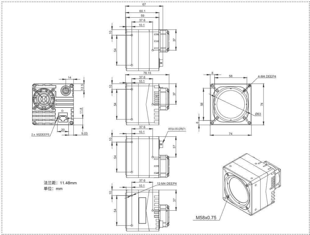
MARS-6500-18GTM/C-NF M58-D1, M58 口 (法兰距 11.48mm)
