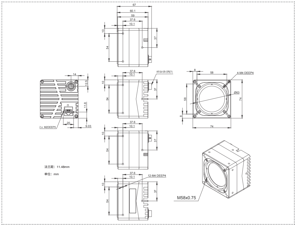
MARS-6501-18GTM/C M58-D1, M58 口（法兰距 11.48mm）
